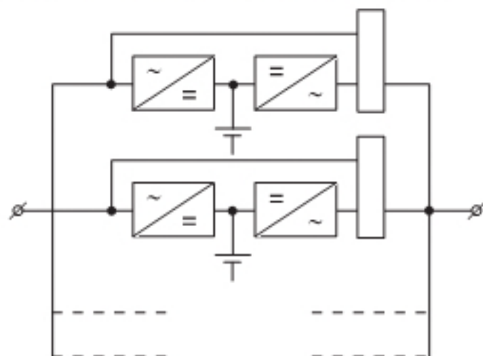
2. Параллельное резервирование N+1
