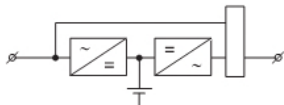
1. Одиночный ИБП
