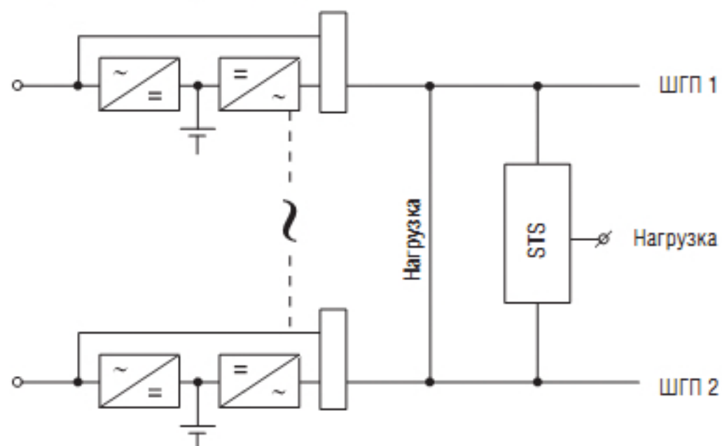
4. Распределенное резервирование
