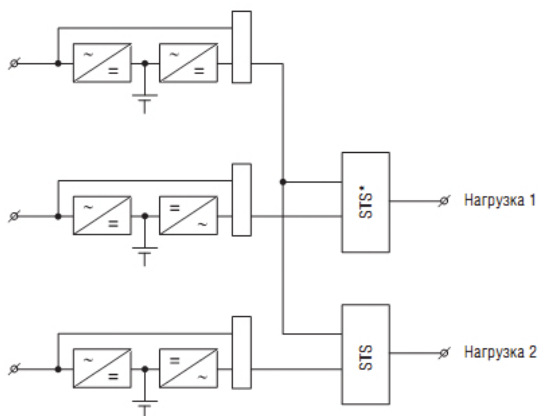
5. Изолированное резервирование N+1
