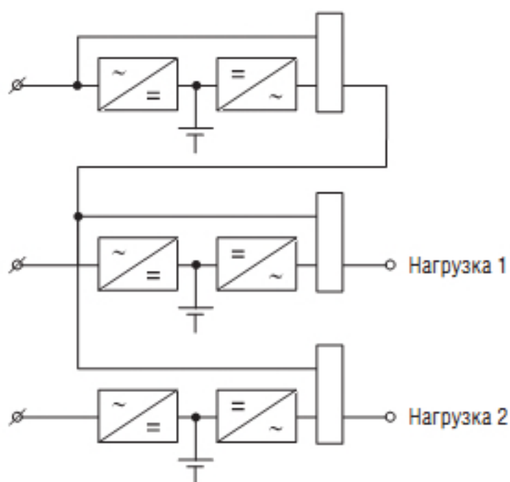
3. Последовательное резервирование N+1
